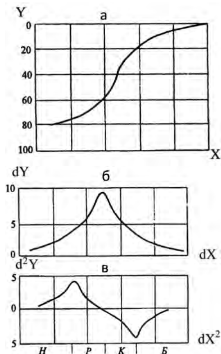
Рис. 1. Логистическая форма зависимости между качеством экосистемы ( Y , в %) и нагрузкой на нее ( X , в усл. ед.) (а), форма зависимости первой производной качества экосистемы от нагрузки на нее с максимумом dY/dX (б), нормирующим зону экологического кризиса K , второй производной d^2Y/dX^2 (в) с максимумом, нормирующим зону экологического риска P , и минимумом, нормирующим зону экологического бедствия B
