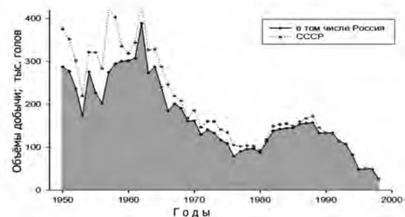
Рис. 1. Промысел морских млекопитающих в СССР во второй половине XX в. (ластроногие и китообразные вместе)
